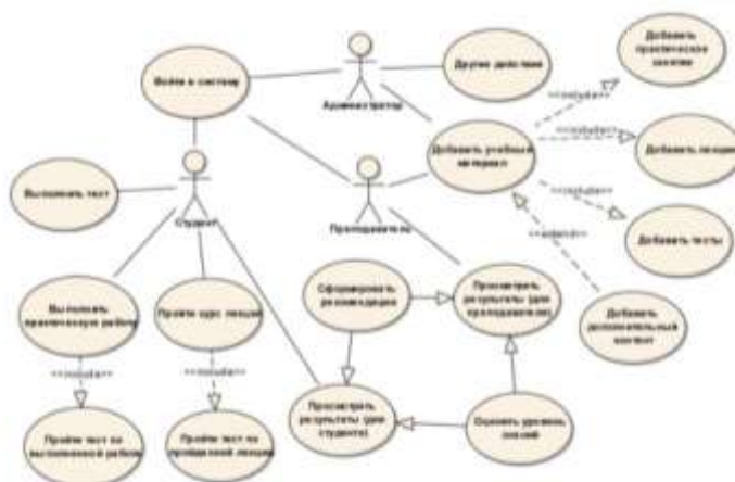
Рис. 4.3 Диаграмма прецедентов
