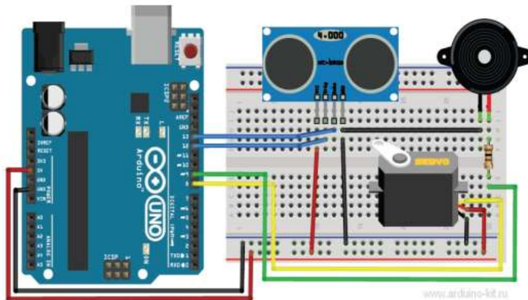
Рисунок 1 – Схема подключения ультразвукового датчика
