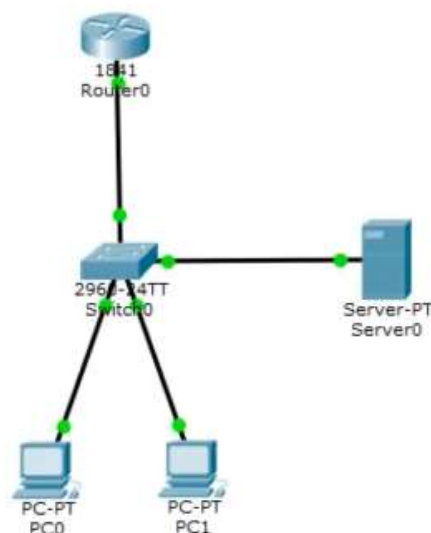
Рисунок 1 – Схема сети
