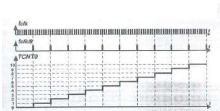
Рис. 1. Работа делителя таймера T0 при коэффициенте делителя 8
