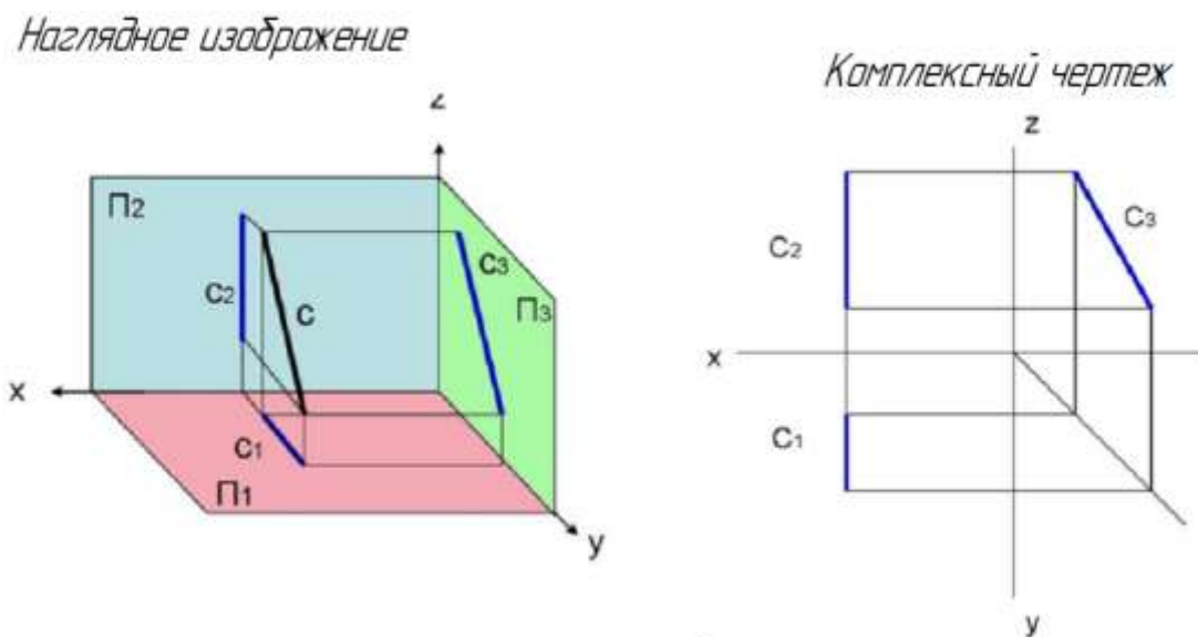
Рис.25 Проекция прямой
