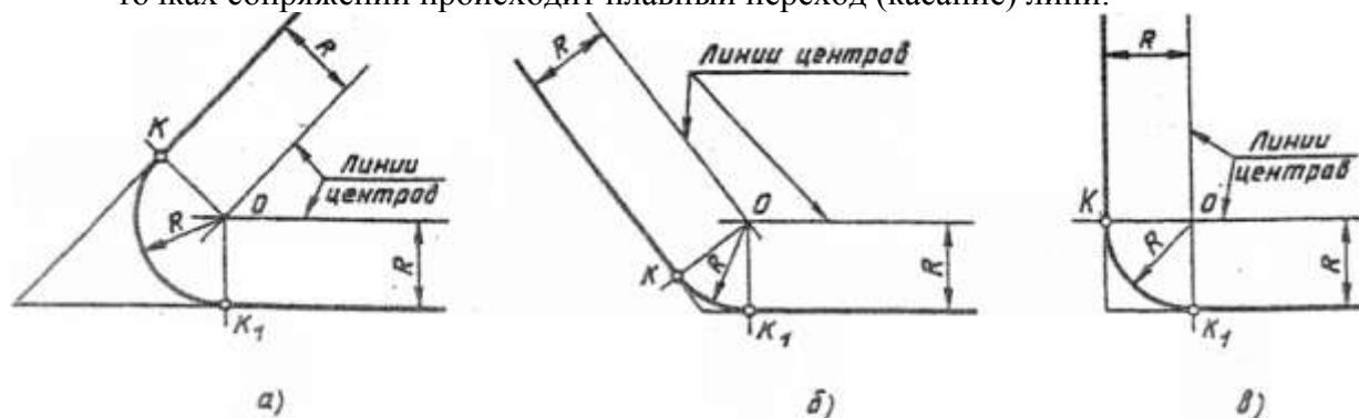
Рис 17 Сопряжение углов
