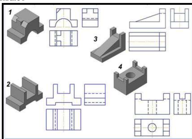
Рис.31 Виды
