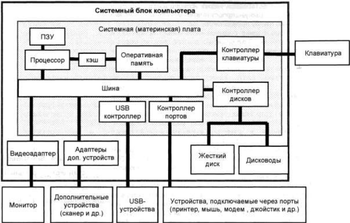
Рисунок 5 – Системный блок
