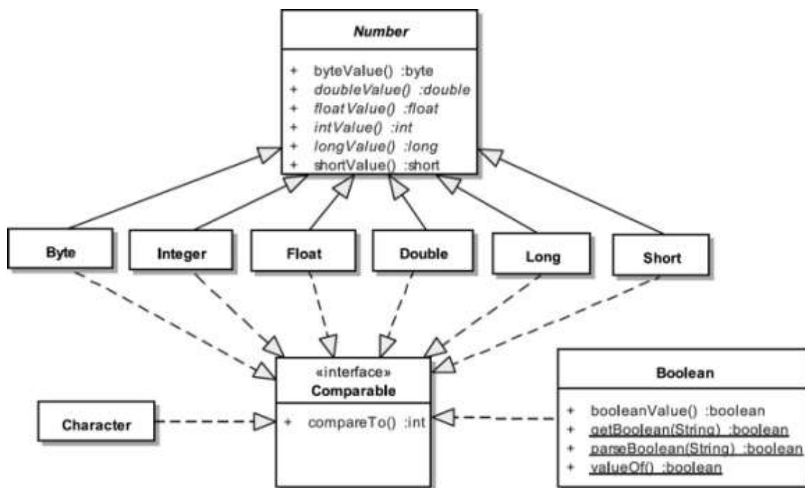
Рисунок 1.2 Иерархия классов-оболочек
