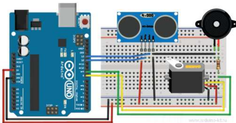
Рисунок 13– Схема сборки
