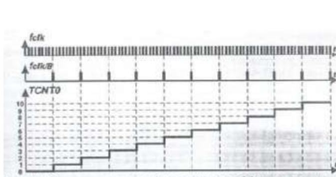
Рис. 1. Работа делителя таймера Т0 при коэффициенте делителя 8
