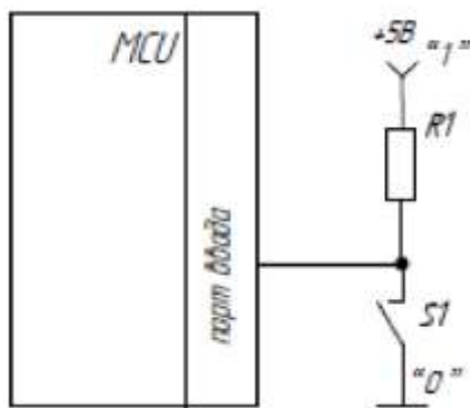
Рисунок 9 – Подключение одиночной кнопки к параллельному порту
