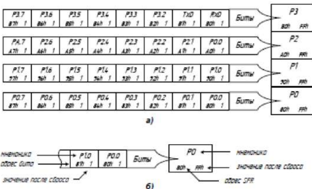
Рисунок 8 – Адреса SFR параллельных портов
