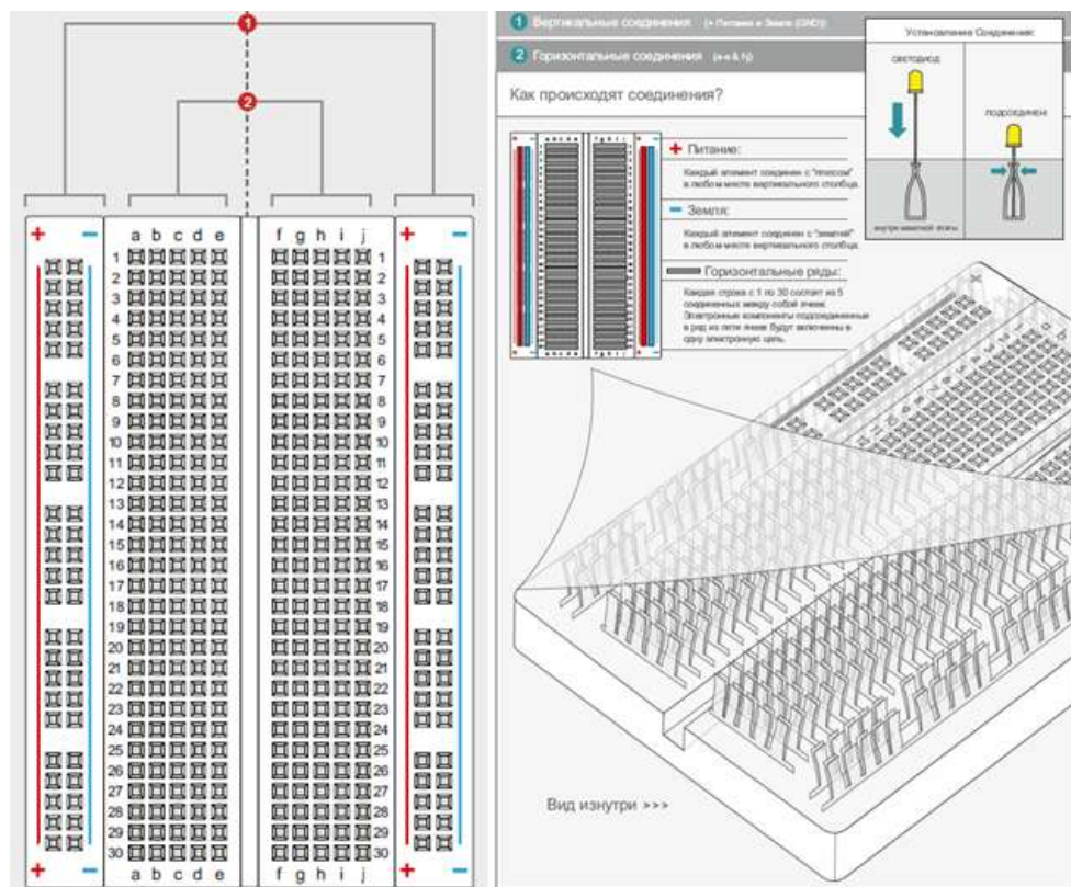
Рисунок 2 – Макетная плата
