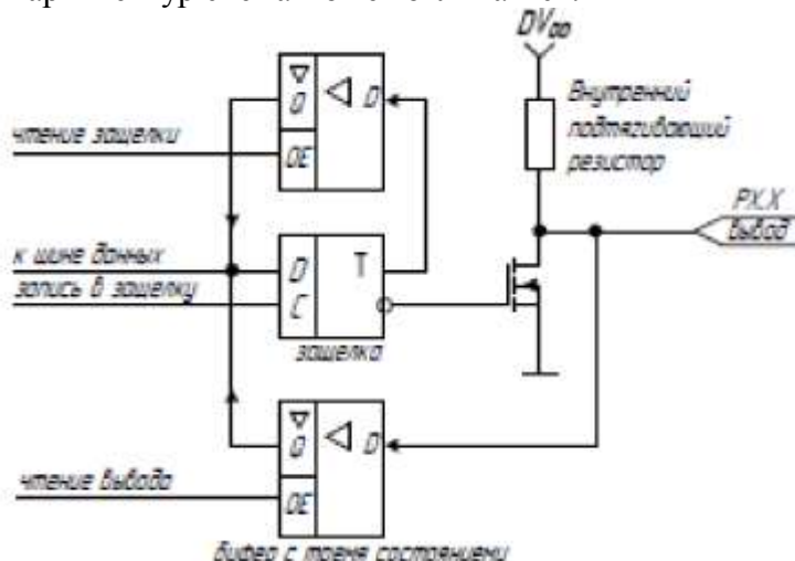
Рисунок 4 – Упрощенная схема одного бита параллельного квазидвунаправленного порта
