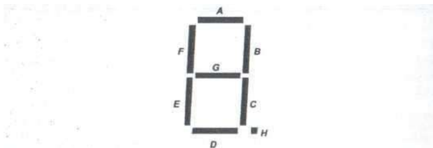
Рис. 1. Внешний вид и структура семисегментного индикатора
