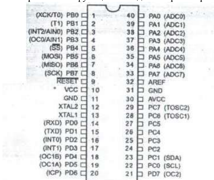
Рис. 1. Расположение выводов микросхемы контроллера АТmega8535 (DIP40)
