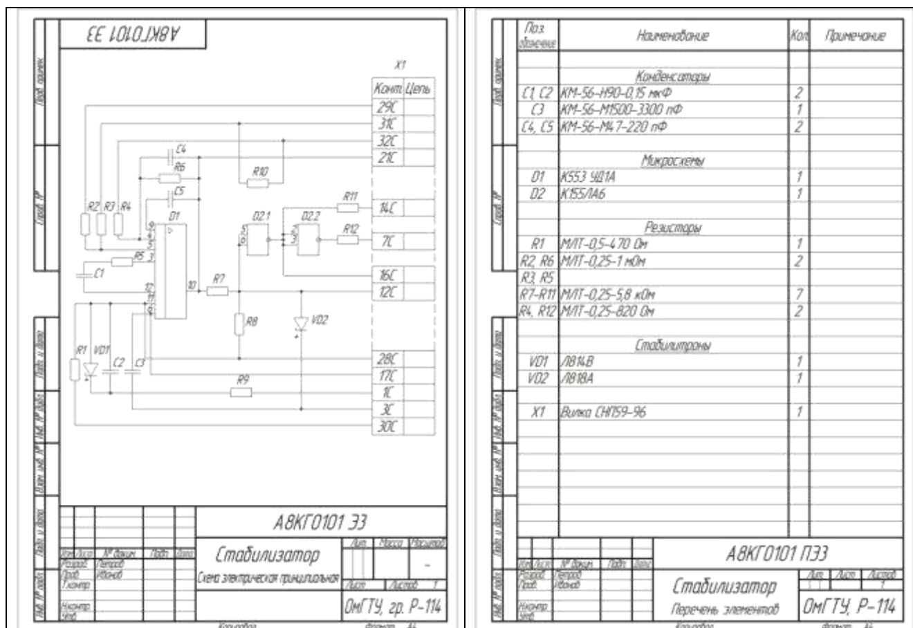
Рис 51 Пример выполнения
