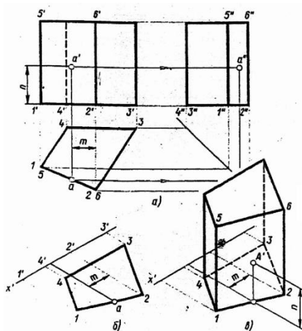
Рис.5 Проекция призмы
