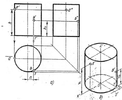
Рис.7 Проекция прямого цилиндра
