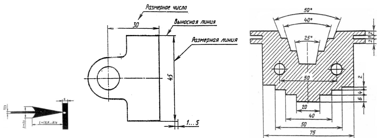
Рис.4 Нанесение размеров
