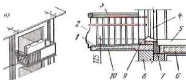
Рисунок 14 - Конструкция балкона
