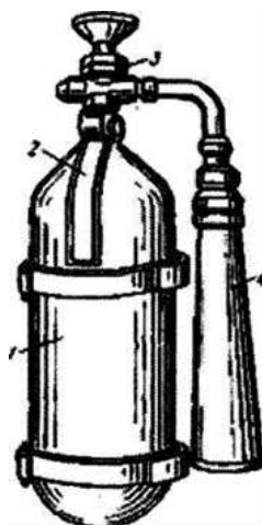
Рис. 2. Огнетушитель ОУ-2: 1 – баллон; 2 – курок; 3 – вентиль; 4 – раструб.
