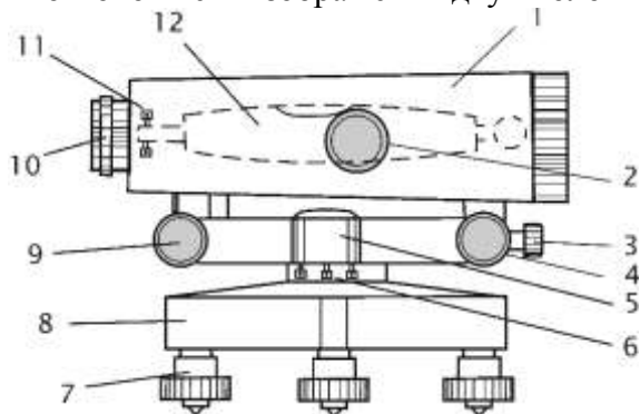
Рисунок 9. Устройство нивелира Н-3:
