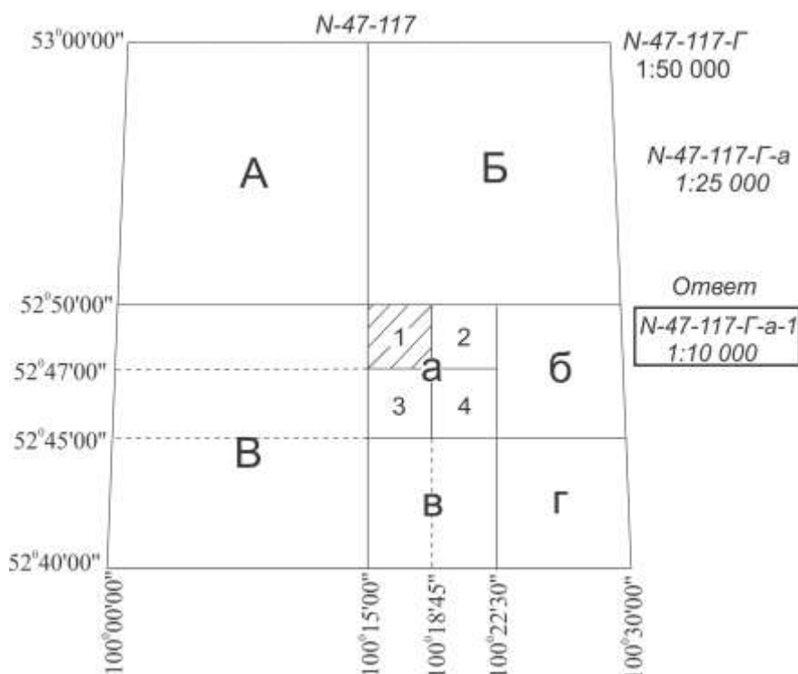
Рис. 3 Определение номенклатуры листов карт
