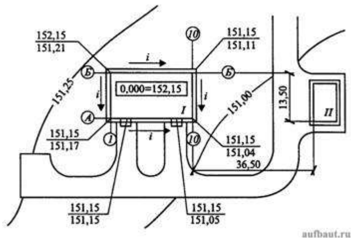
Рисунок 14. Пример выполнения вертикальной и горизонтальной привязок в учебной практической работе: I - проектируемое здание; II - существующее здание; i - направление стока поверхностных вод; A, Б, 1, 10 - обозначения осей
