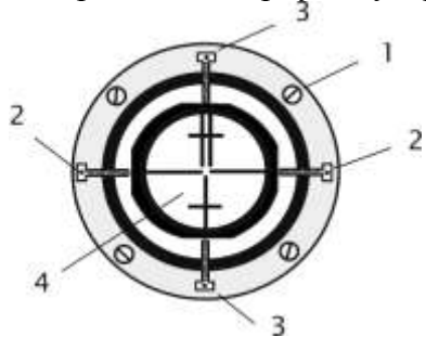
Рисунок 7. Крепление сетки нитей: 1 – крепёжный винт окуляра; 2, 3 – горизонтальные и вертикальные исправительные винты сетки нитей; 4 – сетка нитей.
