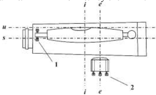
Рисунок 11. Оси и исправительные винты нивелира: ss – визирная ось зрительной трубы; ii – ось вращения прибора; uu – ось цилиндрического уровня; ee – ось круглого уровня; 1 – исправительные винты цилиндрического уровня; 2 – исправительные винты круглого уровня.
