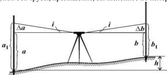
Рисунок 11. Поверка цилиндрического уровня. Измерения из середины
