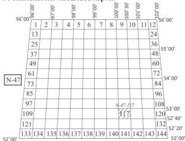
Рис. 8. Определение номенклатуры листа карты масштаба 1: 100 000
