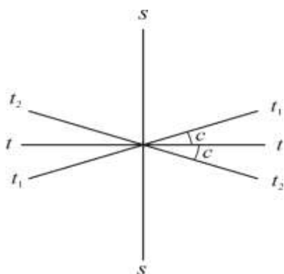
Рисунок 5. Проверка визирной оси: ss – визирная ось; tt – верное положение оси вращения трубы; t_1t_1 , t_2t_2 – положение оси вращения трубы при круге право и круге лево.
