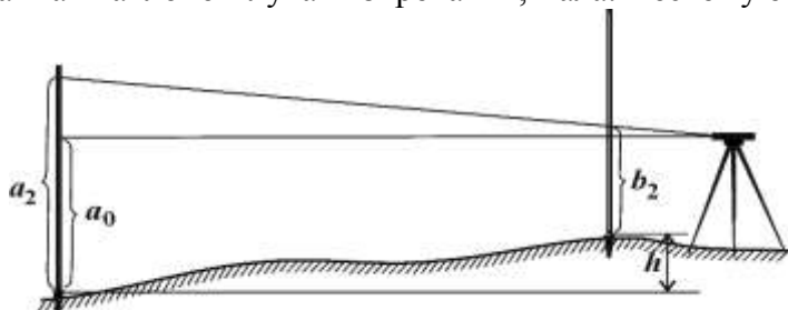
Рисунок 12. Поверка цилиндрического уровня. Измерения с неравными расстояниями до реек
