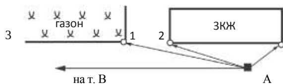
Рис. 12. Абрис тахеометрической съемки
