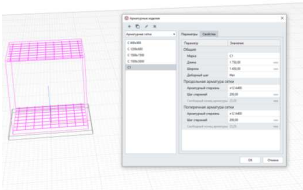
Рисунок 2.3 – Арматурные изделия
