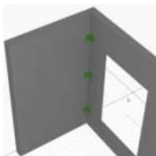
Рисунок 10.5 - Размещение закладных. Ответные закладные. Панель шахты лифта со всеми закладными. Общий вид
