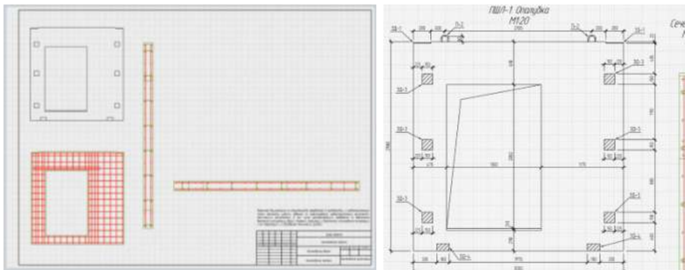
Рисунок 10.13 - Чертеж. Все виды. Готовая опалубка
