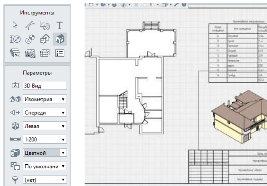
Рисунок 8.5 - Добавление аксонометрии модели здания.
