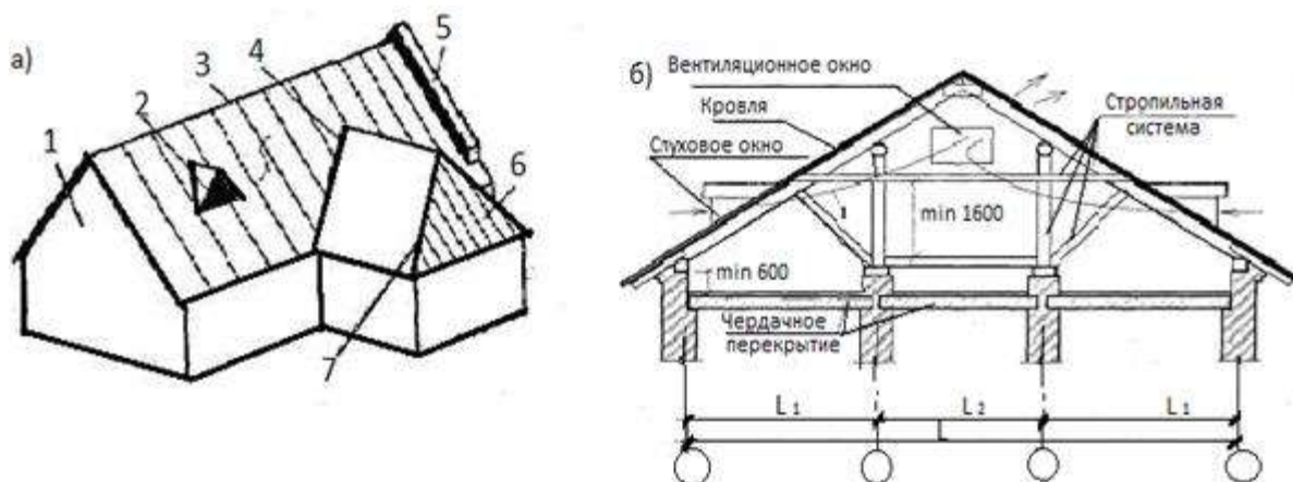
Рисунок 4.1 – Задание на выполнение скатной кровли а - общий вид: 1 — фронтон; 2 — слуховое окно; 3 — конек; 4 — ендова; 5 — щипец; 6 — вальма; 7 — ребро; б –поперечное сечение;
