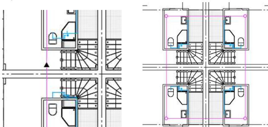
Рисунок 9.2 – Симметричная привязка
