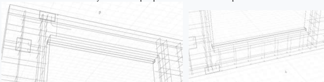
Рисунок 10.8 - Ручное армирование зоны под проемом. Копирование стержней
