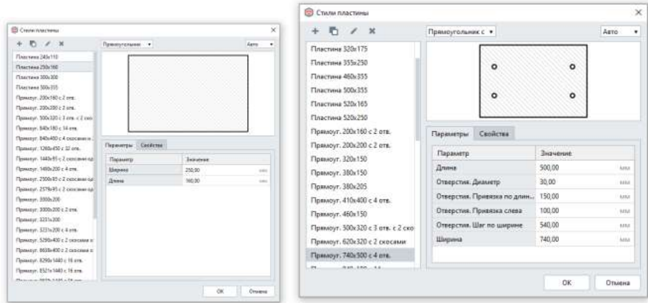
Рисунок 3.3 Стиль пластины опорной плиты
