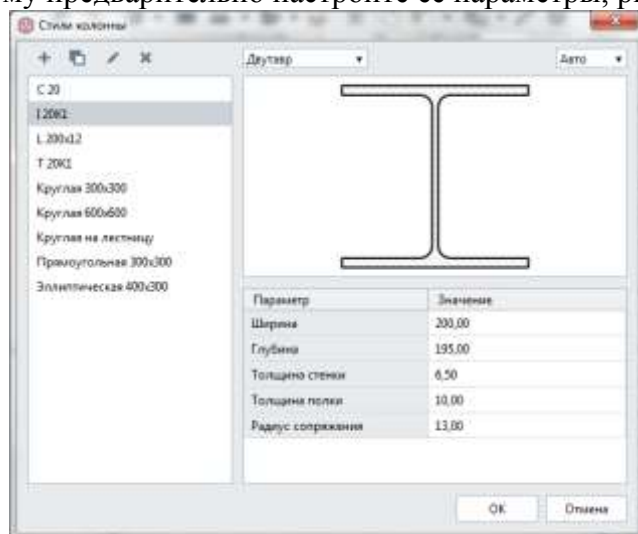
Рисунок 3.1 – Параметры колонны
