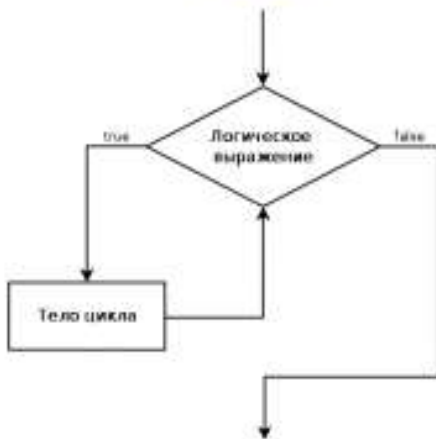
Цикл while
