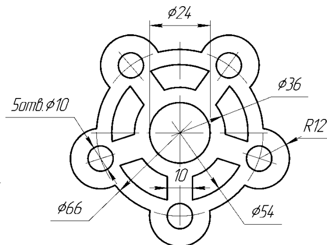
Прокладка
