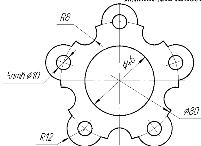
Прокладка
