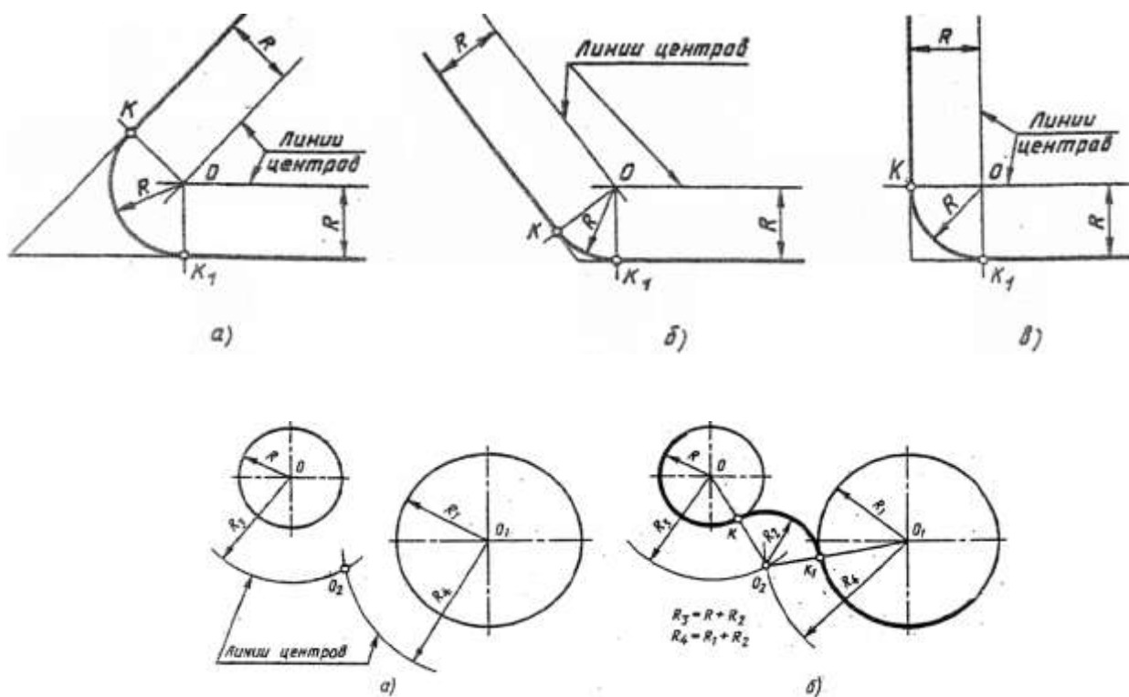
Рис.18 Внешнее касание
