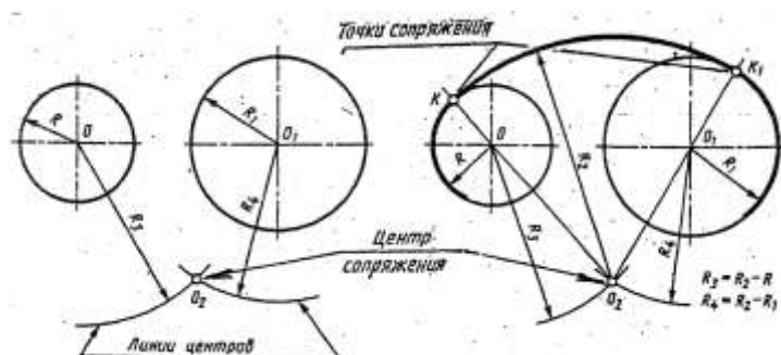
Рис.19 Внутреннее касание
