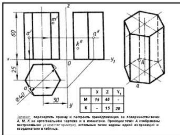
Рис.11 Проекция шестигранной правильной
