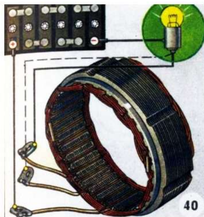
Рисунок 15 Проверка обмотки статора на обрыв
