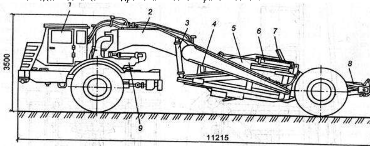
Рис. 5. Скрепер ДЗ-11П:
