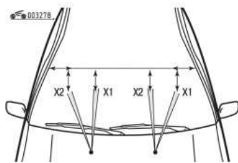
Рисунок 1 Регулировка жиклеров стеклоомывателей ветрового стекла
