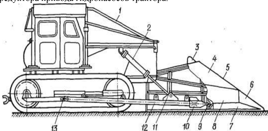
1 — ограждение; 2 — гидроцилиндр; 3 — козырек; 4 — наклонный щит; 5 — отвал; 6 — нож-колун; 7 — боковые ножи; 8 — вертикальный щит; 9 — гнездо; 10 — съемная шаровая головка; 11 — упорная стойка; 12 - универсальная толкающая рама; 13 — опора рамы
