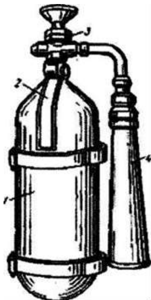
Рис. 2. Огнетушитель ОУ-2:
