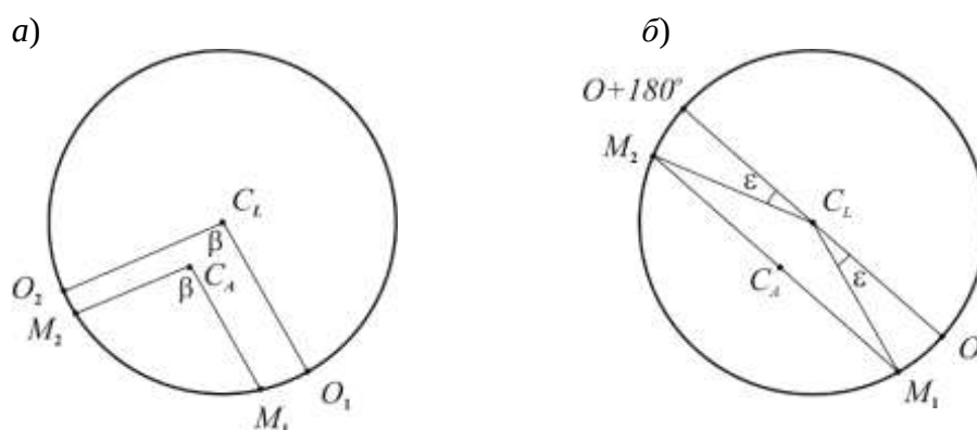
Рисунок 4. Эксцентриситет алидады: а – влияние на результат измерения угла; б – исключение влияния; C_L – центр лимба; C_A – ось вращения алидады.
