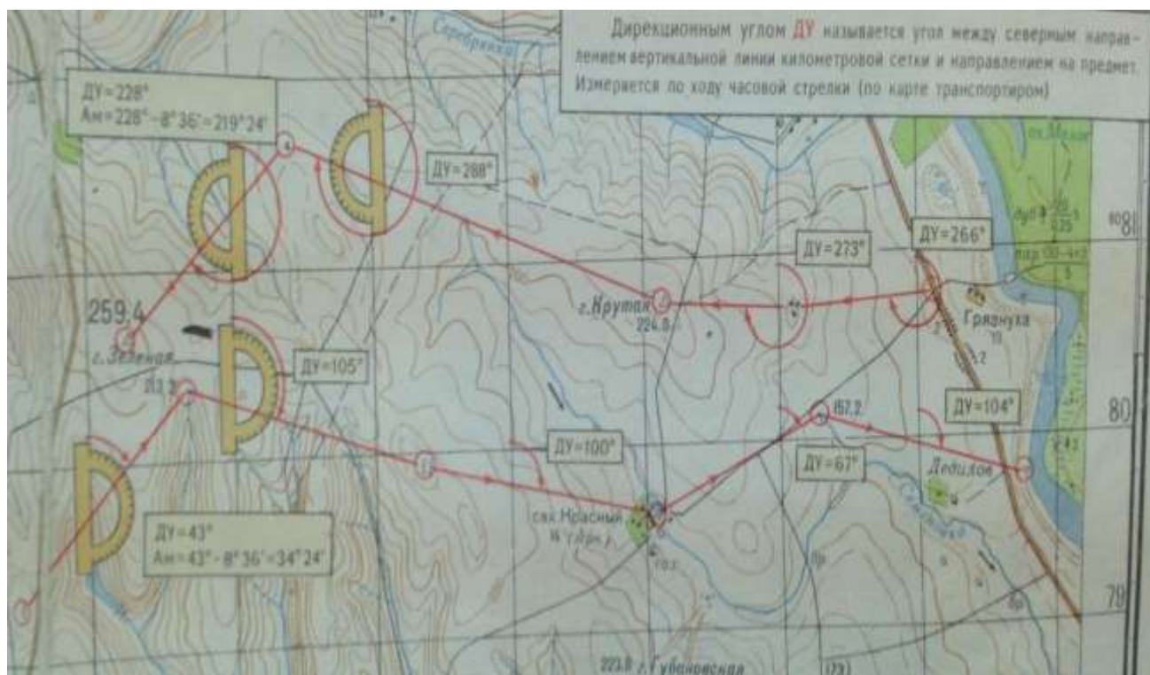
Рис. 13. Измерение дирекционного угла транспортиром
