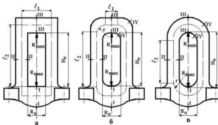
Рисунок 10 – Схема нагружения станины
