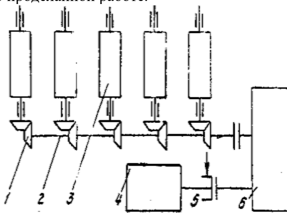
Рисунок 11 – Привод рольганга
