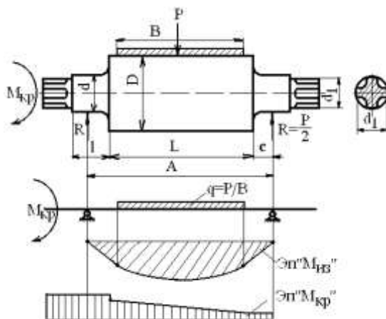
Рисунок 9 – Схема нагружения прокатного валка
