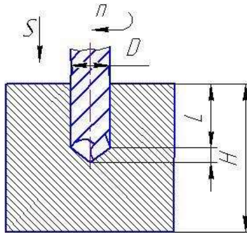
Рисунок 1 – Эскиз обработки
