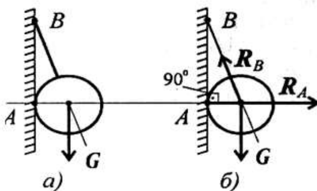
Рисунок 2 - Определение реакции нити и гладкой опоры
