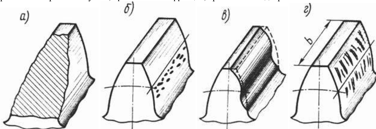
Рисунок. Виды разрушения зубьев
