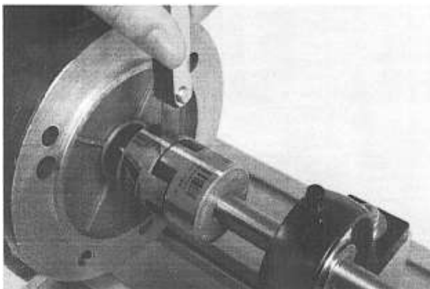
Зазор в положении на 12 часов: 0.95 мм
