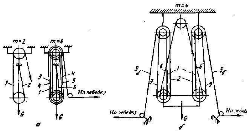
Рисунок 1.6 - Схемы полиспастов
