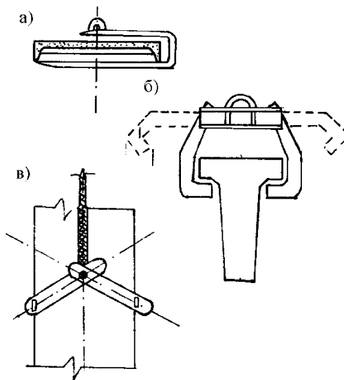
Рис. 3. Беспетлевые захваты
