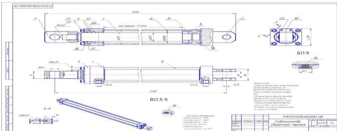
Рисунок 1 – Конструкции гидроцилиндров промышленного оборудования
