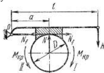
Рисунок 6 - Расчетная схема одноколодного тормоза
