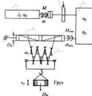
Рисунок 1 – Кинематическая схема механизма подъема
