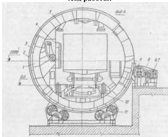
Рисунок 8 – Схема стационарного роторного вагоноопрокидывателя
