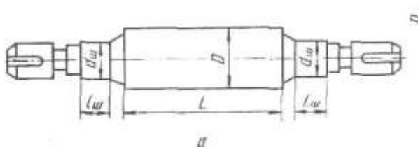
Рисунок 11 – Прокатный валок
