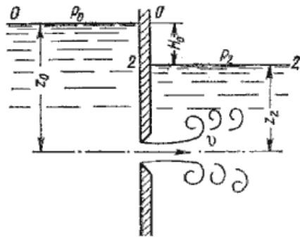
Рисунок 2 - Истечение под уровень
