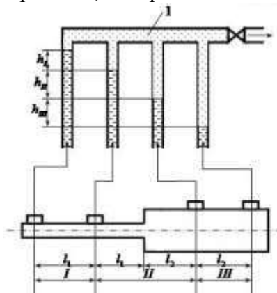
Рисунок -1. Измерение разности напоров на местном сопротивлении. 1-блок дифференциальных пьезометров; l_I, l_{II} –длины участков I и II; l_1, l_2 –длины участка II непосредственно перед и после внезапного расширения; h_I, h_{II}, h_{III} , - потери напоров на участках I, II, III.
