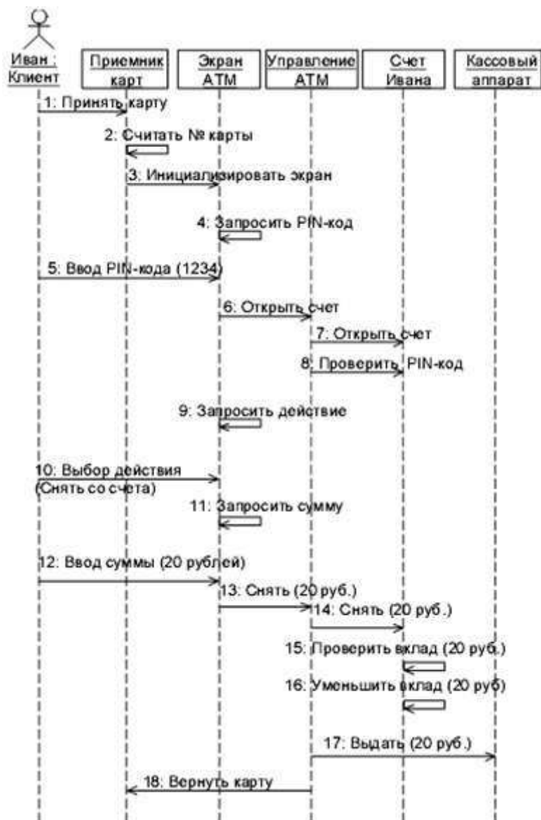
Рисунок 1 – Пример диаграммы последовательности
