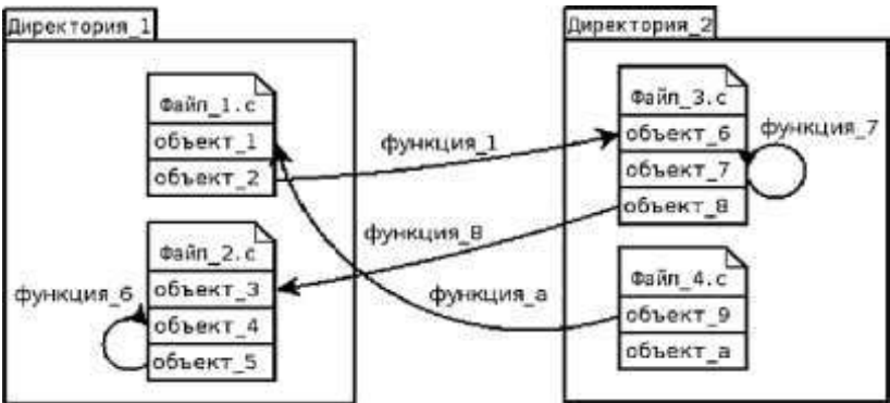
Рисунок 2 – Отображение связей между объектами
