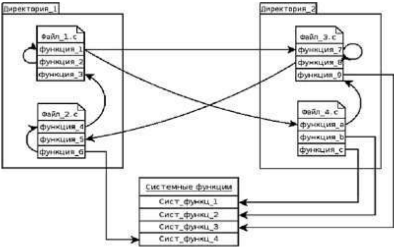
Рисунок 1 – Отображение функциональных связей
