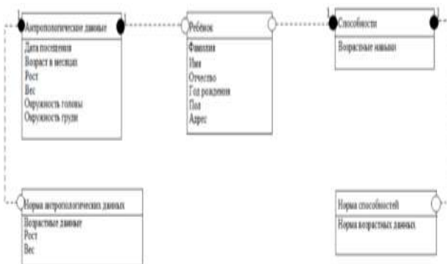
Рис.4.2. Информационная модель
