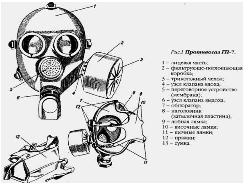
Рисунок 2- Противогаз ГП-7
