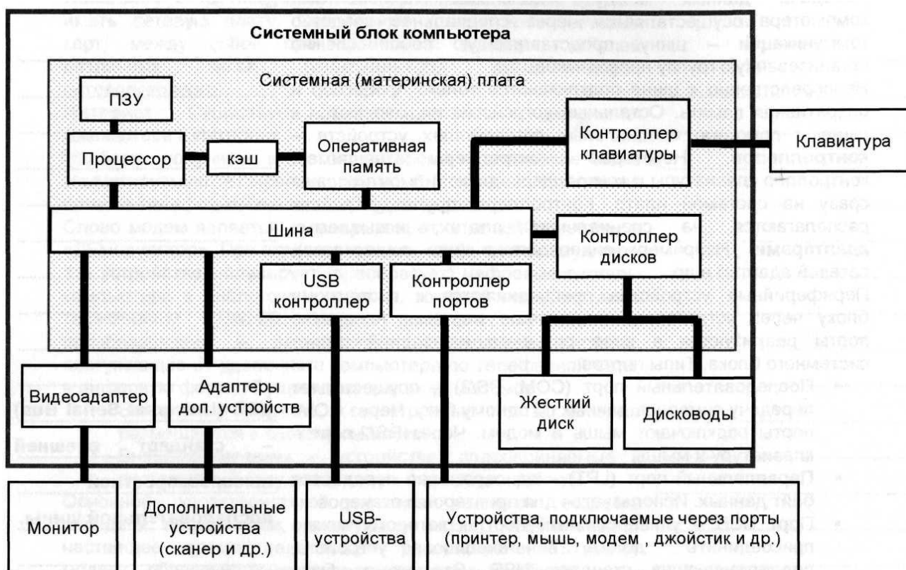
Рисунок 4 – Системный блок
