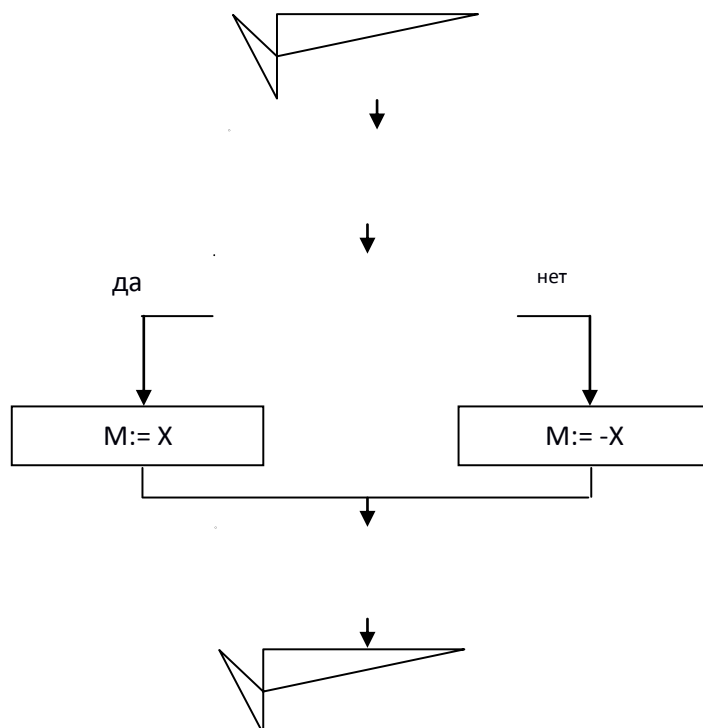
Рисунок 5 – Разветвляющийся алгоритм
