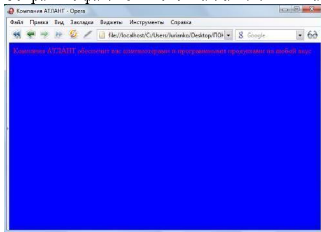
Рис. 1.1 Созданная WEB-страница
