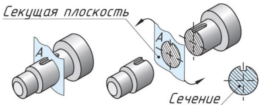
Рисунок 38 Образование сечений
