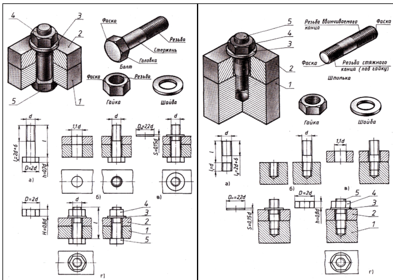
Рис.46 Соединение болтом и шпилькой
