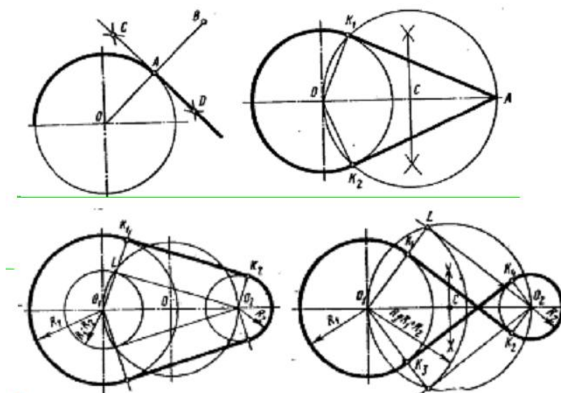
Рис. 15 Построение касательных к окружности.
