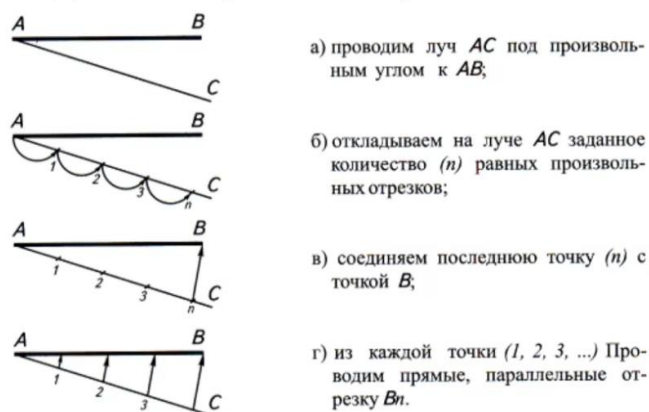
Рис 14 (б) Деление отрезка равные отрезки
