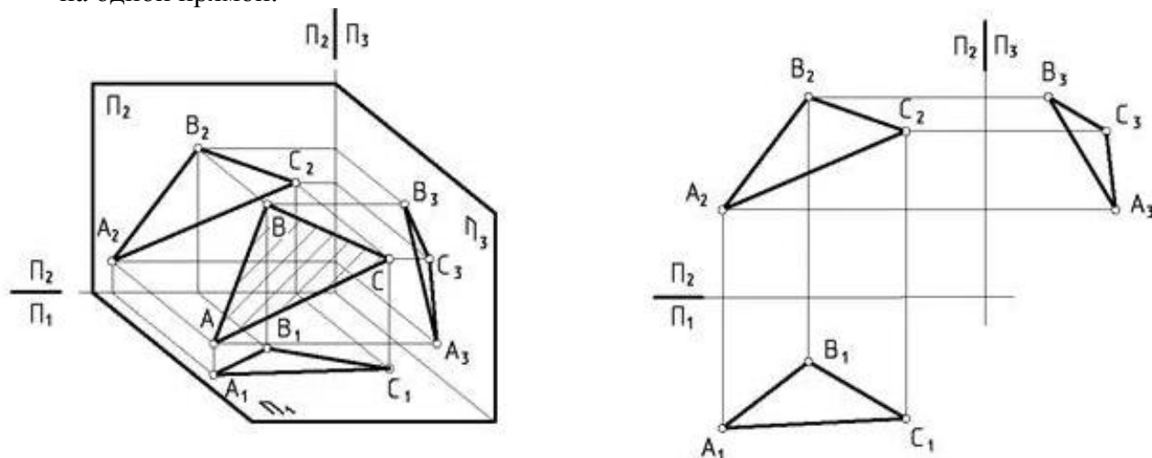
Рис.26 Проекции плоскости
