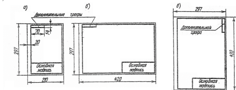
Рис.1 Расположение основной надписи на листе
