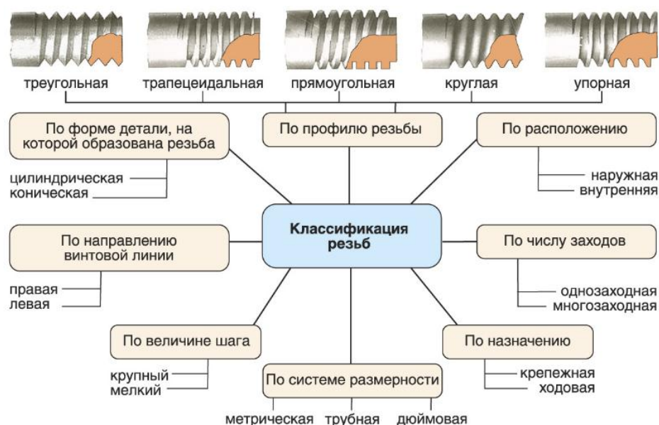
Рис.41 Классификация резьбы
