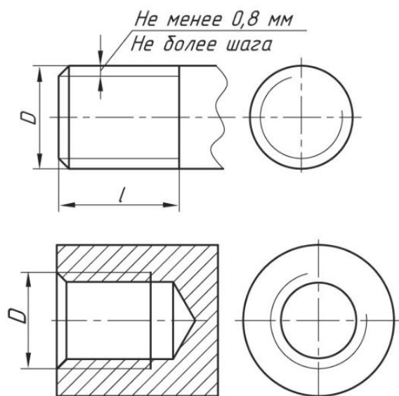
Рис 43 Изображение внешней и внутренней резьбы
