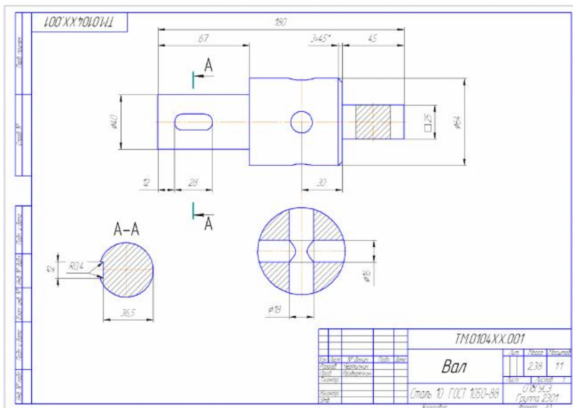
Рис 40 Пример выполнения чертежа
