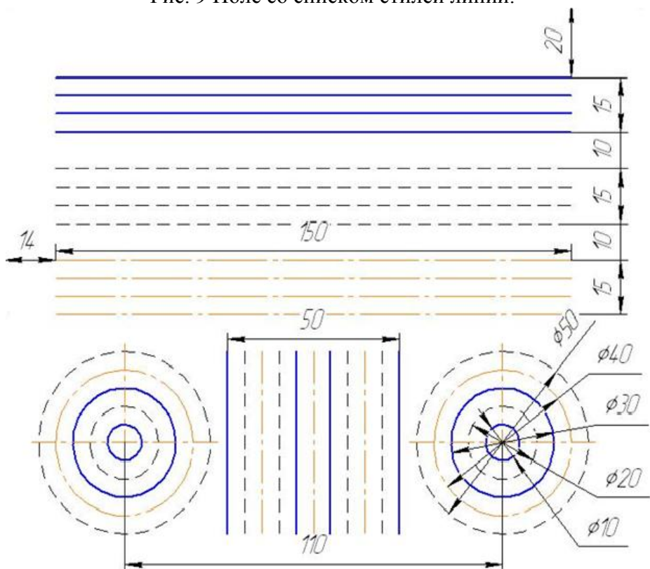
Рис. 10 Линии чертежа
