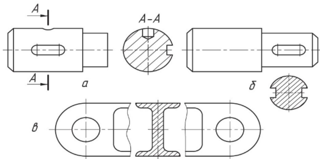
Рис 39 вынесенные сечения
