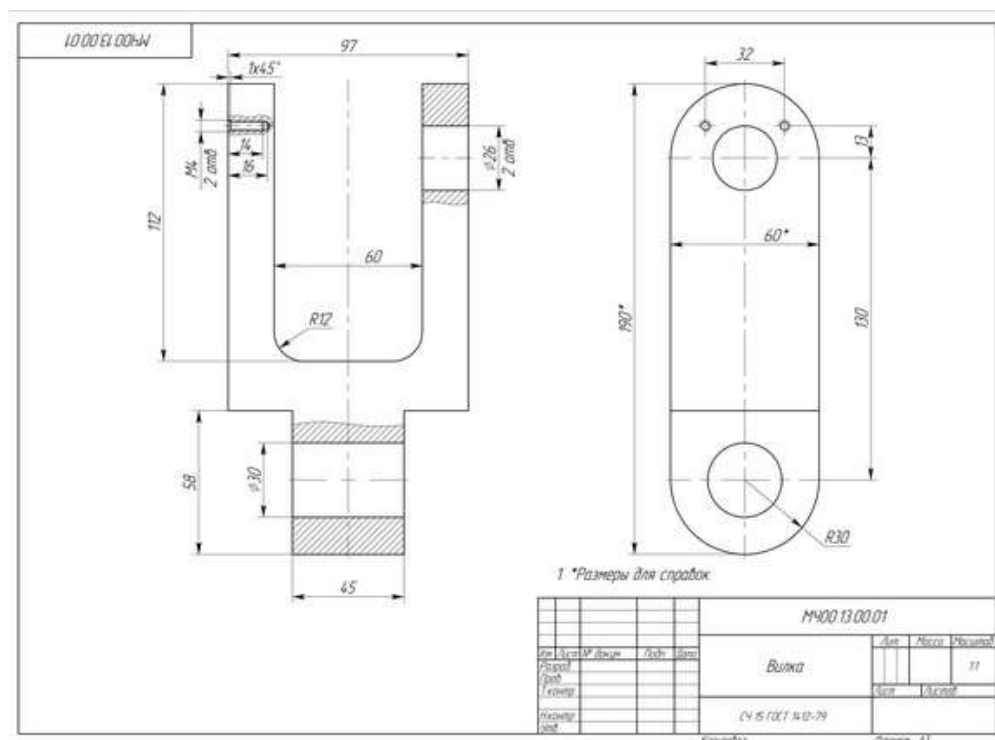
Рисунок 1 – Чертеж детали «Вилка»
