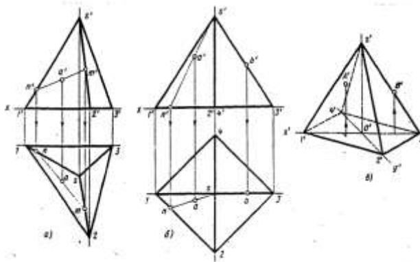
Рис. 6 Проекция пирамиды
