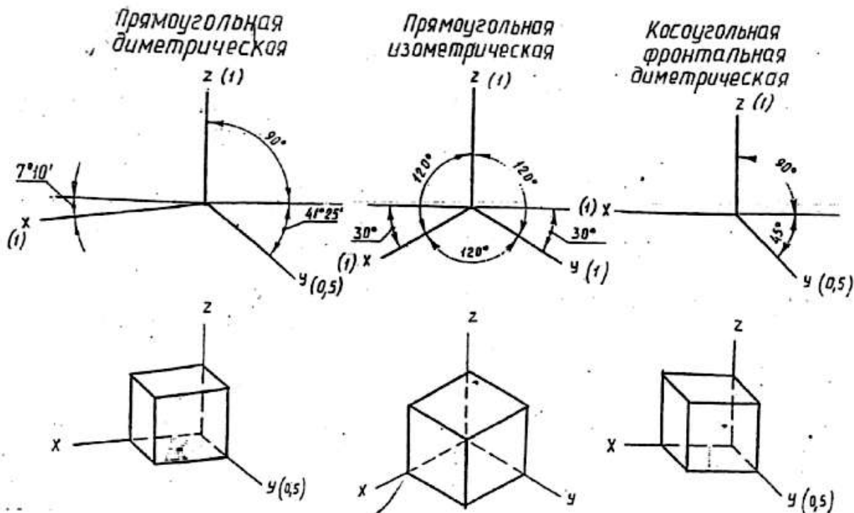
Рис.12 Виды аксонометрических проекций
