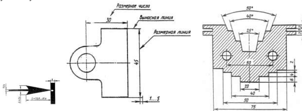
Рис.4 Нанесение размеров
