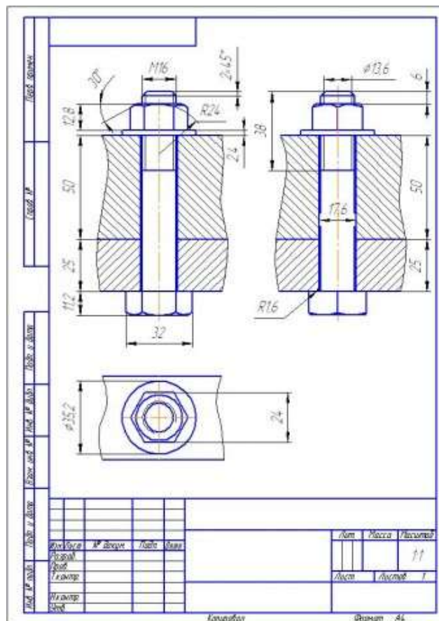
Рис.28 Пример выполнения чертежа болтового соединения
