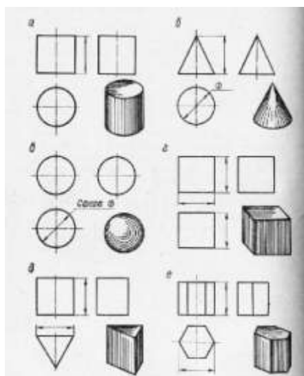
Рис.9 Проекции геометрических тел
