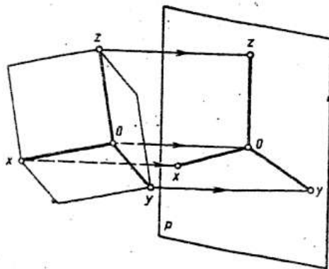
Рис.11 Направление проецирующих лучей в аксонометрии
