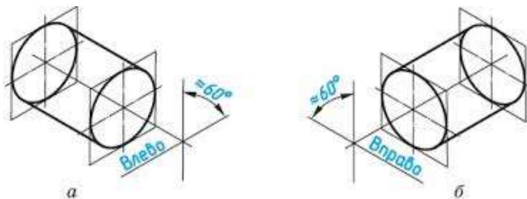
Рис.15 Аксонометрия цилиндрической поверхности
