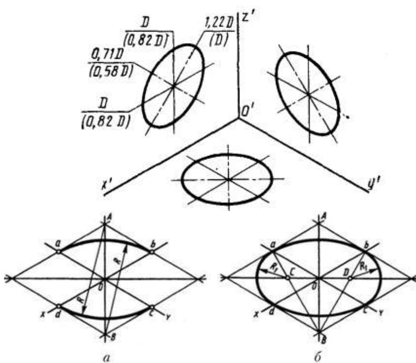
Рис.14 Аксонометрия окружности
