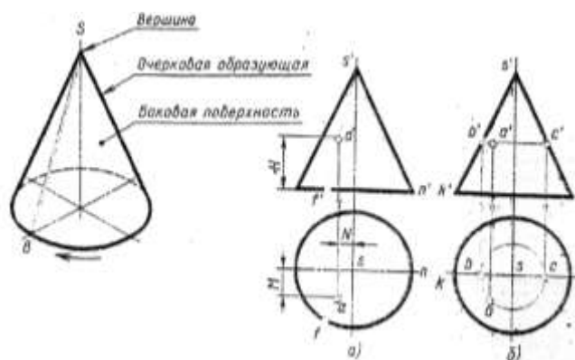
Рис.8 Проекции конуса
