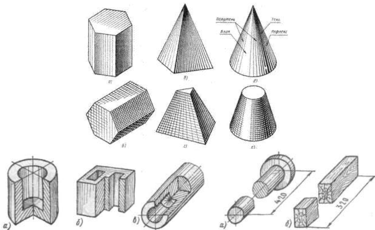
Рис.31 Типы наглядных изображений геометрических поверхностей и контуров технических деталей
