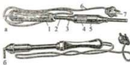
Рисунок 3- Электрические паяльники
