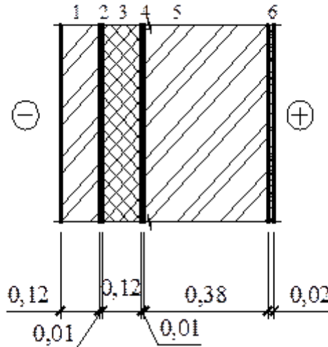
Рисунок 1 – Эскиз стены
