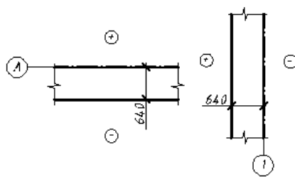
Рисунок 3 - Привязка наружных самонесущих стен
