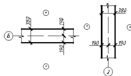
Рисунок 4 - Привязка внутренних стен
