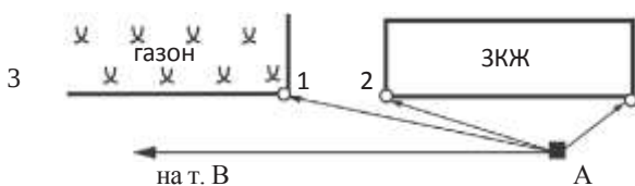
Рис. 12. Абрис тахеометрической съемки
