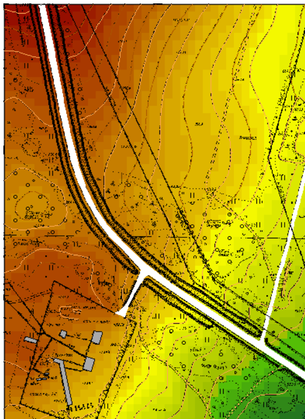
Рис. 18. Изображение матрицы с размером элемента 10 м
