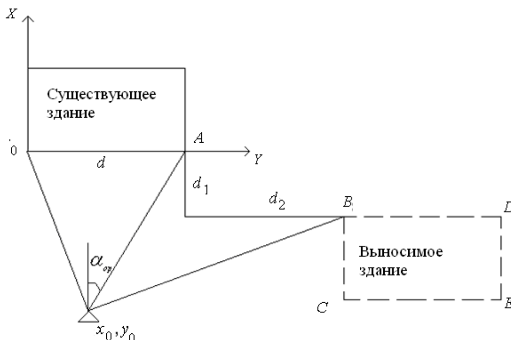
Рисунок 48. Вынос проекта здания в натуре у от существующего с помощью тахеометра.
