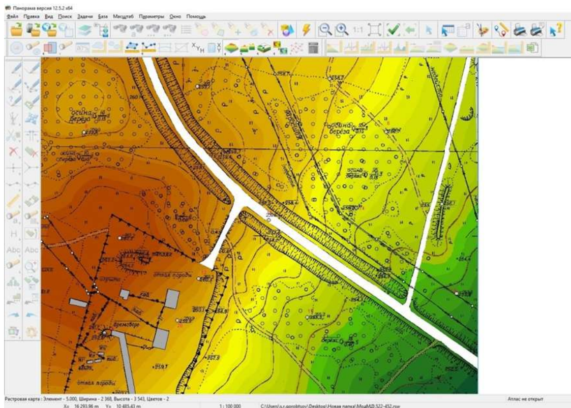
Рис. 13. Изображение ЦМР в виде TIN
