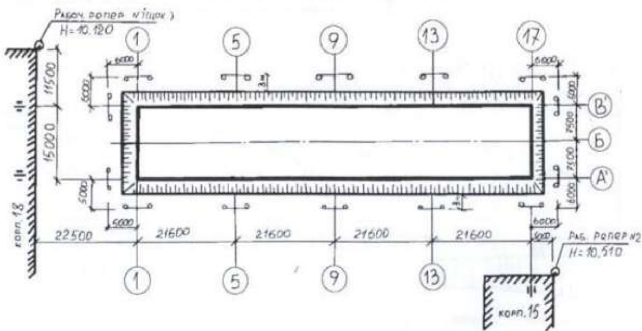
Рисунок 49 Исполнительная схема разбивки осей здания.
