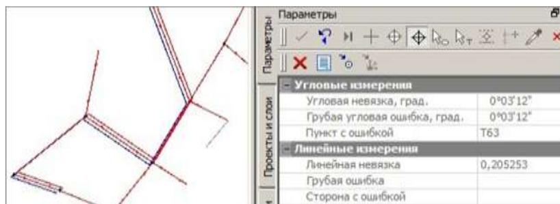
Рис. 21 Построение цепочки
