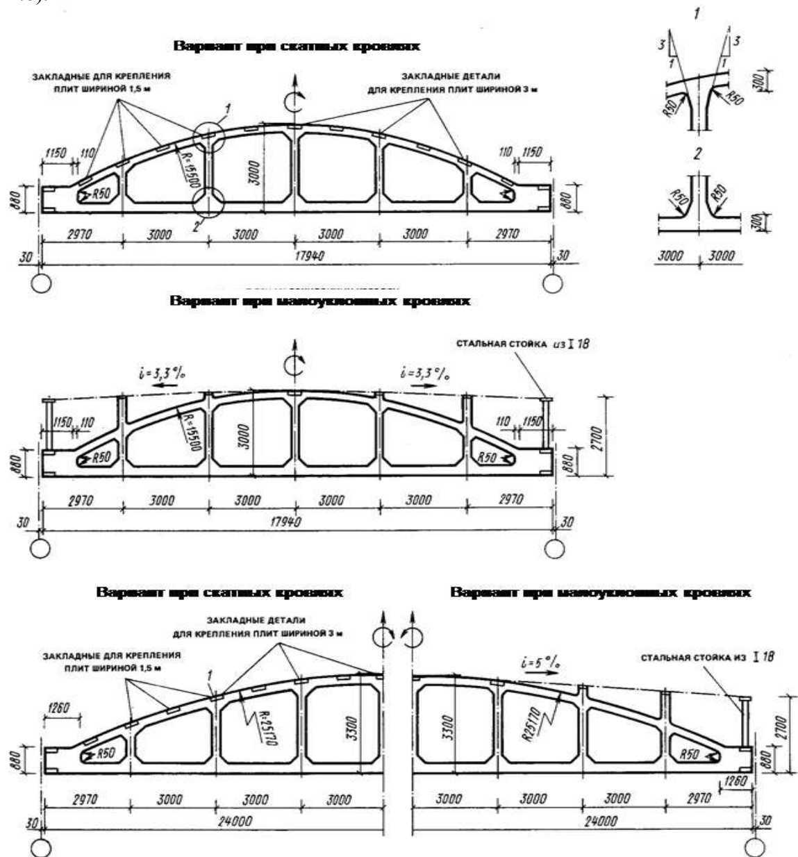
Рис. 4.8. Стропильные фермы (проекты 18 и 24 м)
