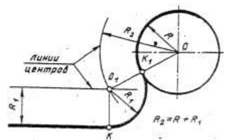
Рисунок 13- Смешанное касание
