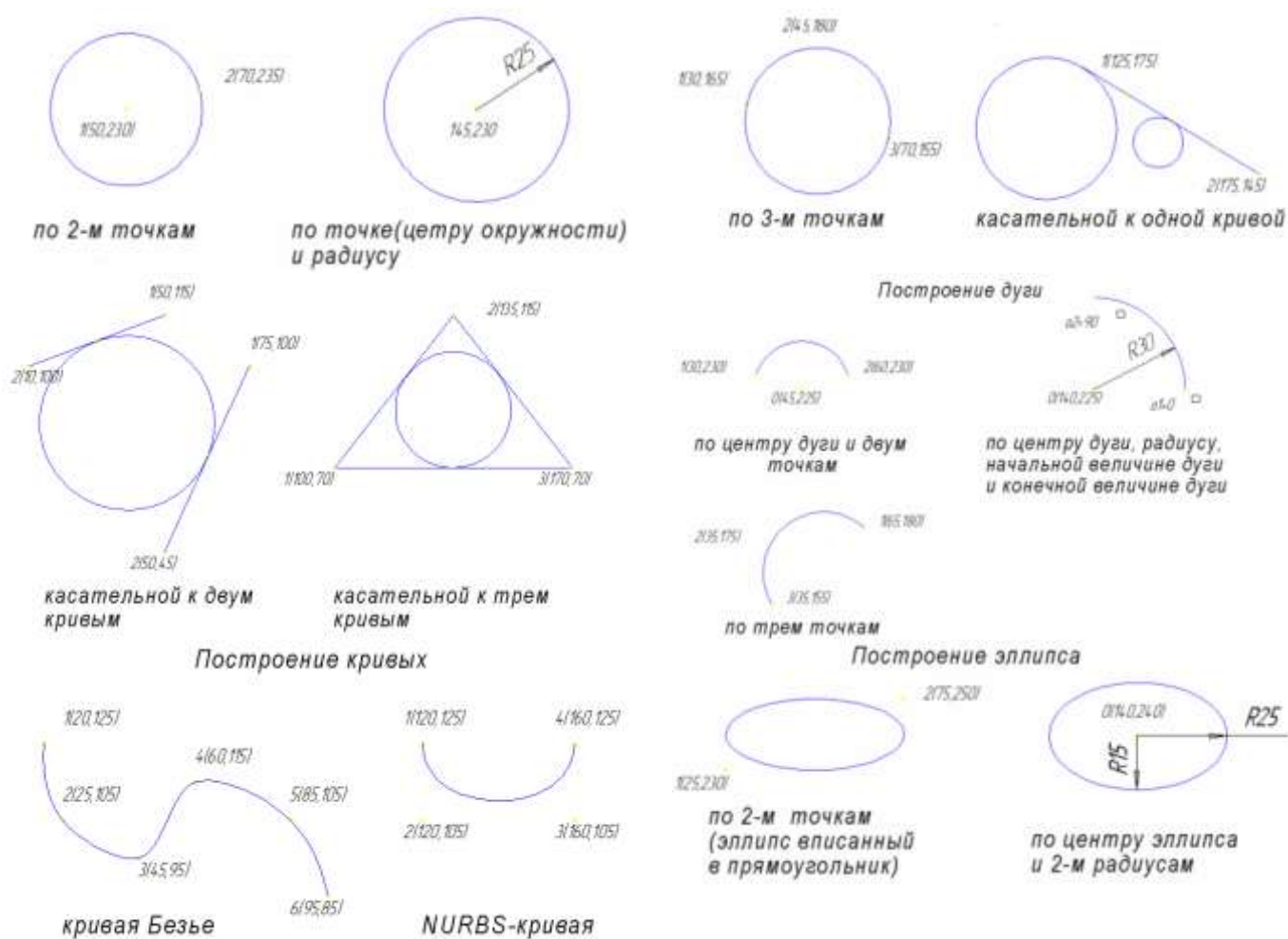
Рисунок 36 - Сопряжение
