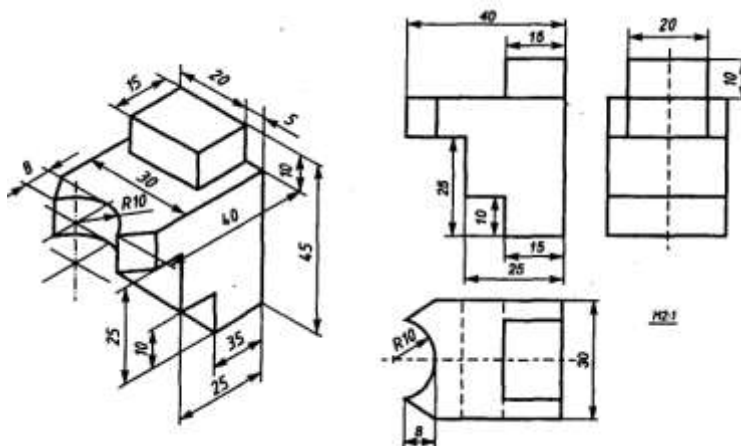
Рисунок 37 – Чертеж детали
