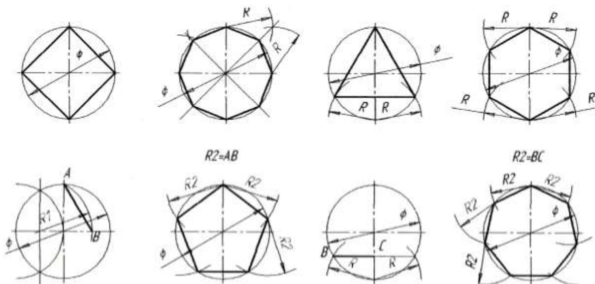
Рисунок 8 - Деление окружности на равные части:
