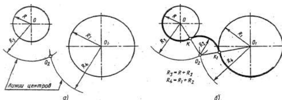
Рисунок 11 - Внешнее касание
