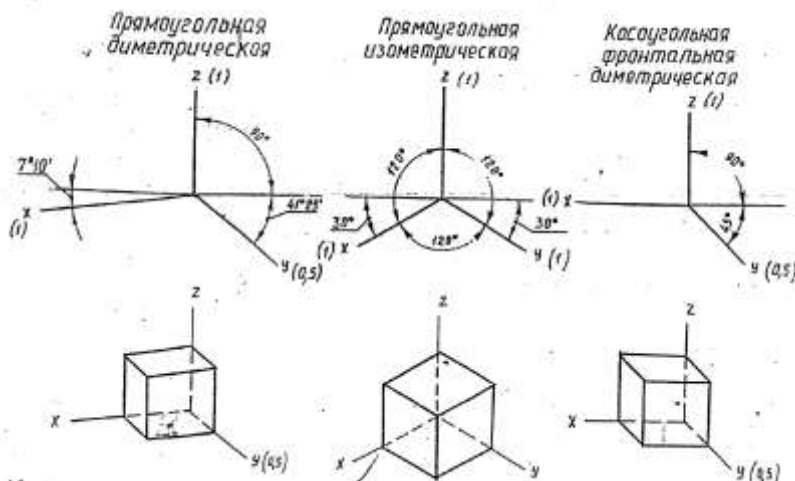
Рисунок 20 - Виды аксонOMETрических проекций
