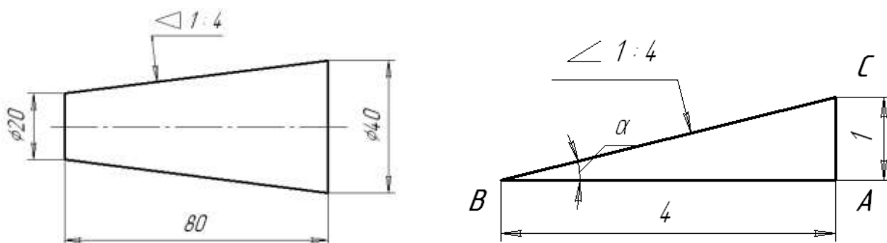
Рисунок 9 – Построение конусности, уклона
