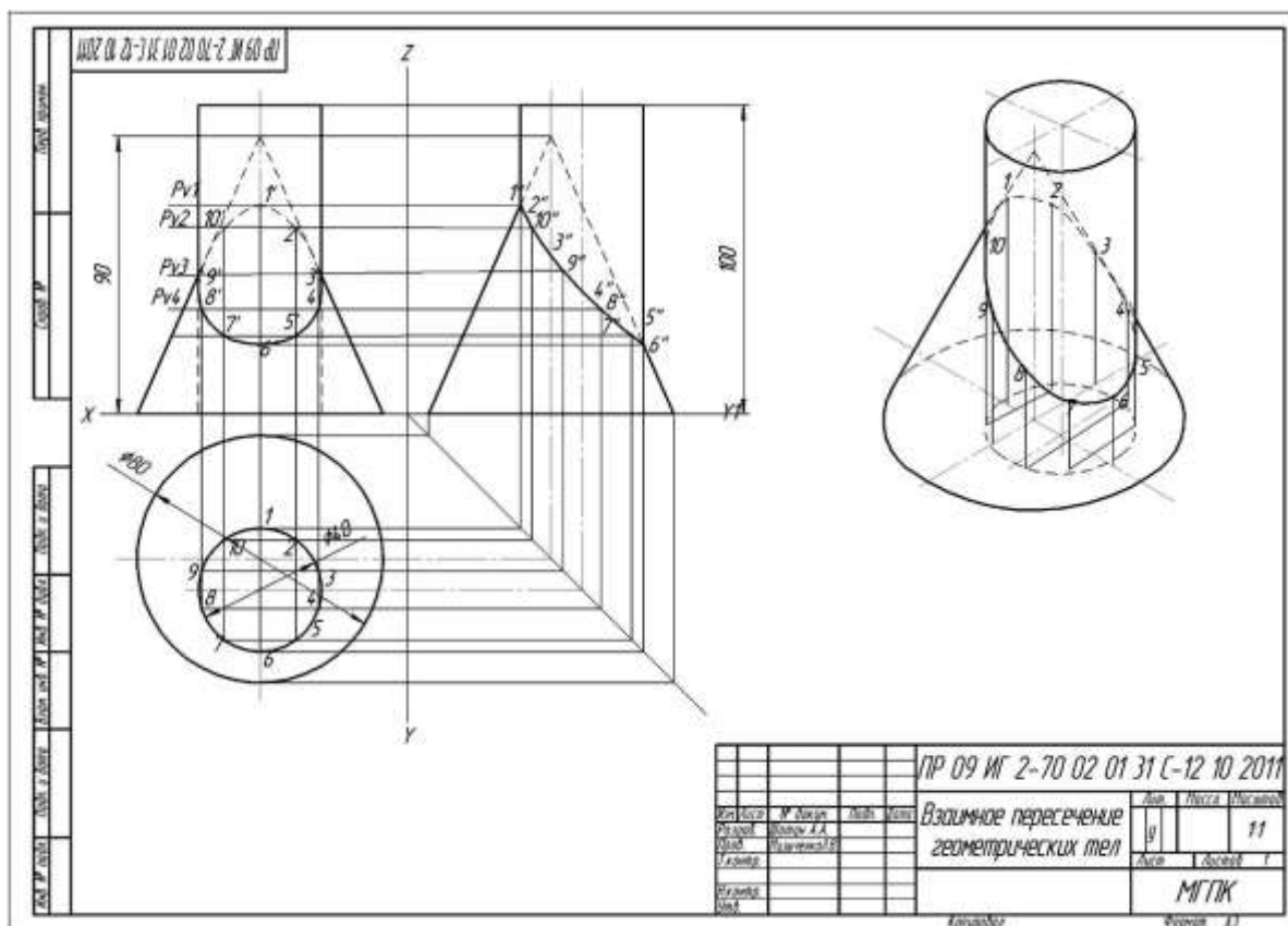
Рисунок 30 – Пример оформления графической работы
