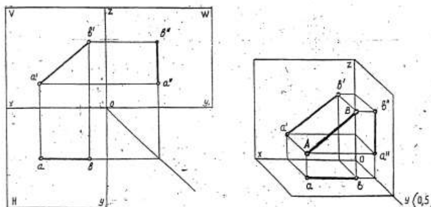
Рисунок 15 - Проекции прямой
