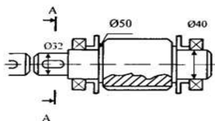
Рисунок 10- Ведомый вал
