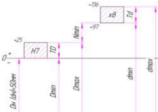
Рис.1 Схема расположения полей допусков соединения \frac{H7}{\text{Æ}50 \text{ x}8} .
