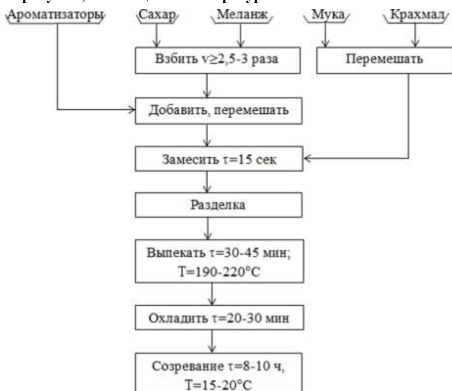
Рисунок 4 – Технологическая схема приготовления бисквита основного
