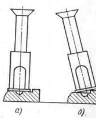
Рисунок 4 - Положение лупы при измерении отпечатка: а — правильное положение б — неправильное положение
