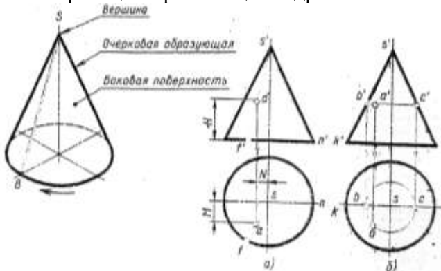
Рис.9 Проекция конуса
