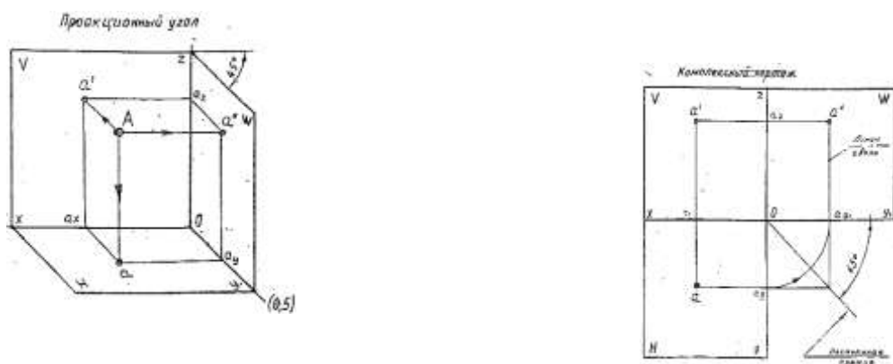
Рис.4 Проекция точки
