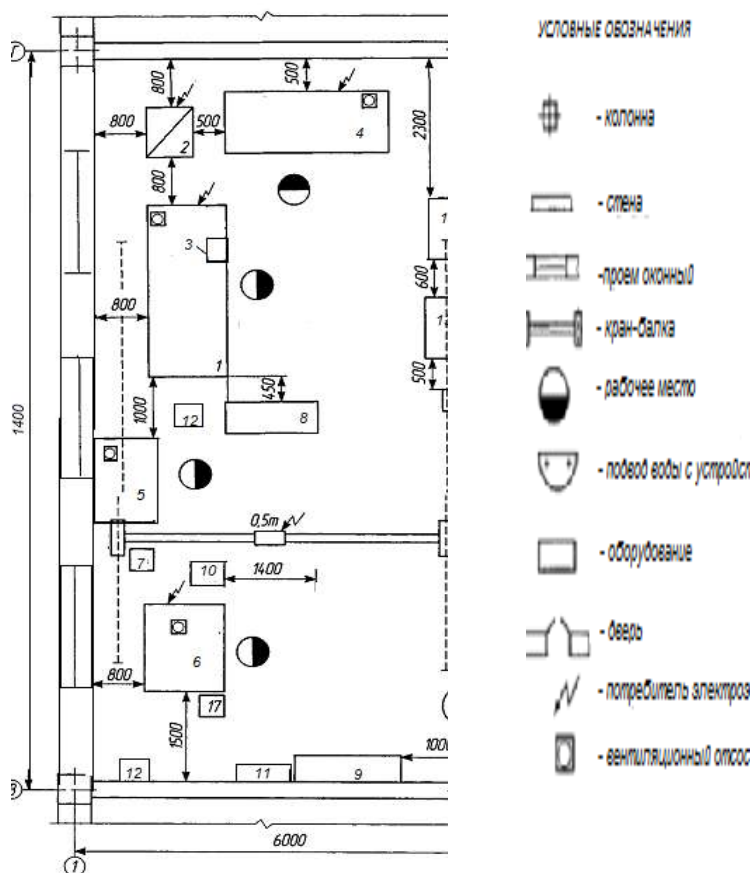
1 - Токарно-винторезный станок 16K20
