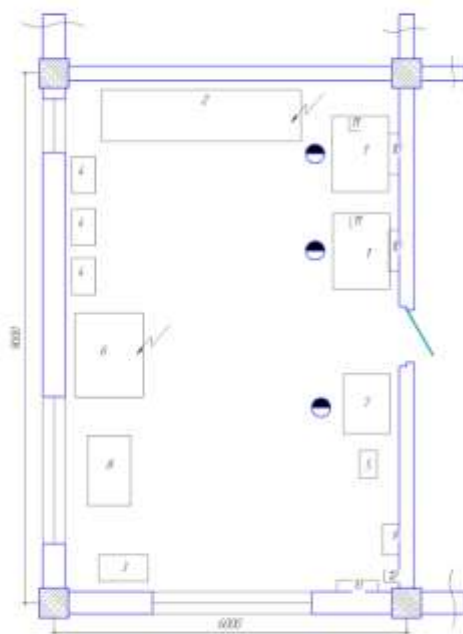
Планировочное решение слесарно-механического участка
